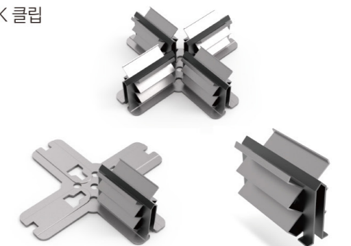
MZK클립 고정부위 모자이크패널 시공
